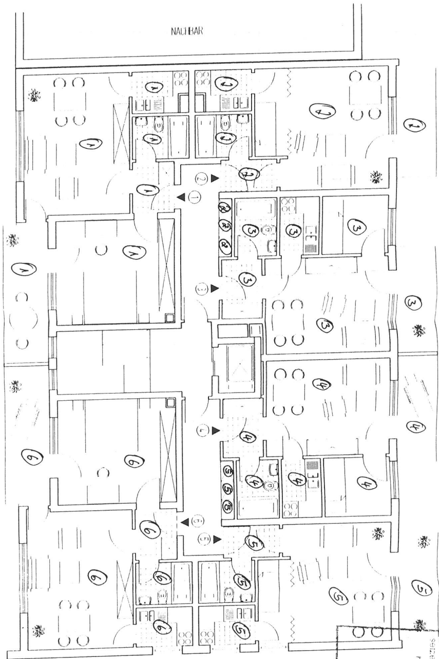
1. OBERGESCHOSS M 1:100
